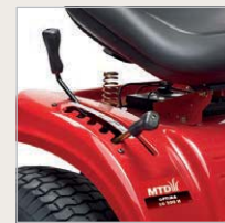
MANUAALINEN LEIKKUKORKEU- DEN SÄÄTÖ SEKÄ LEIKKUPÖYDÄ KYTKENTÄ
